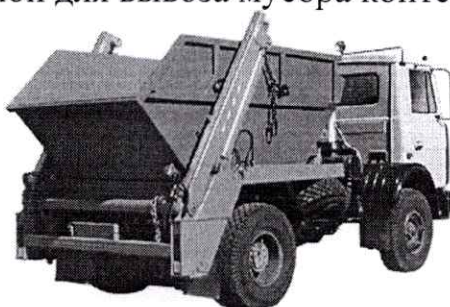
Рис. 4.16. Бункеровоз МКС-3501 на шасси МАЗ-5551А2
