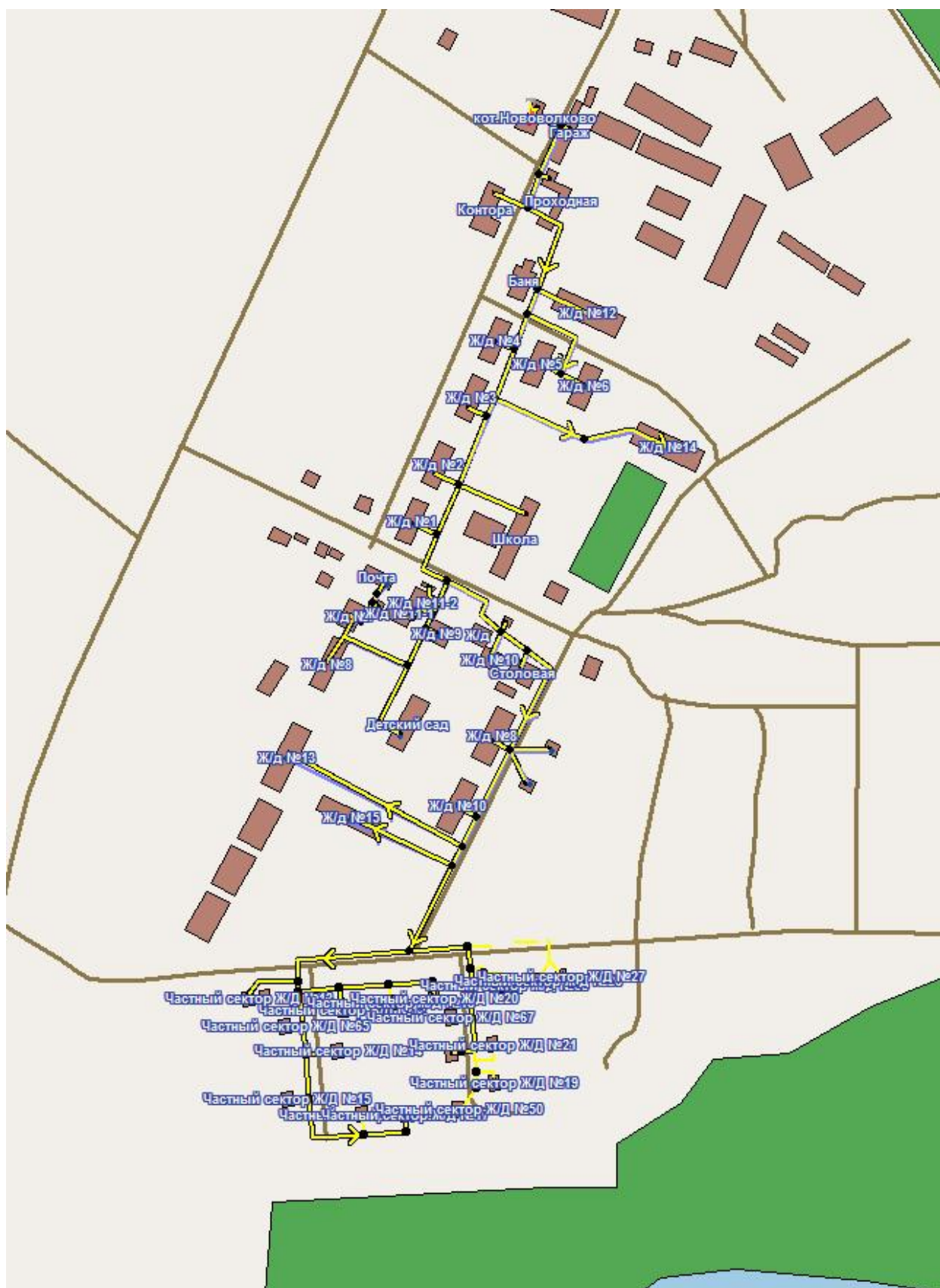
Рисунок 3.1 - Схема тепловой сети котельной д. Нововолково
