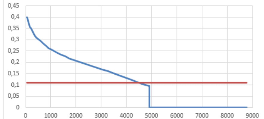
Рисунок 2.7 - График Россандера котельной д. Ивойлово
