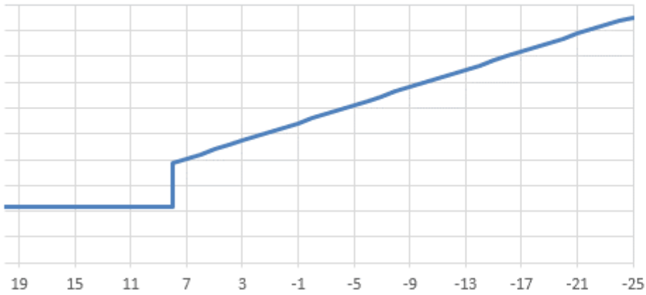
Рисунок 2.5 - График Россандера с. Покровское ДОХБ
