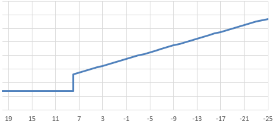
Рисунок 2.4 - График Россандера котельной д. Нововолково
