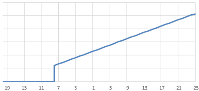
Рисунок 2.9 - График Россандера котельной д. Городище
