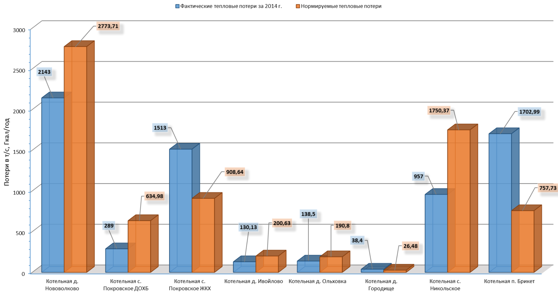
Рисунок 3.10 - Потери в тепловых сетях котельных сельского поселения Волковское
