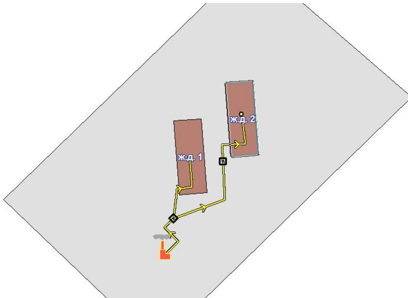
Рисунок 3.6 - Схема тепловой сети котельной д. Городище
