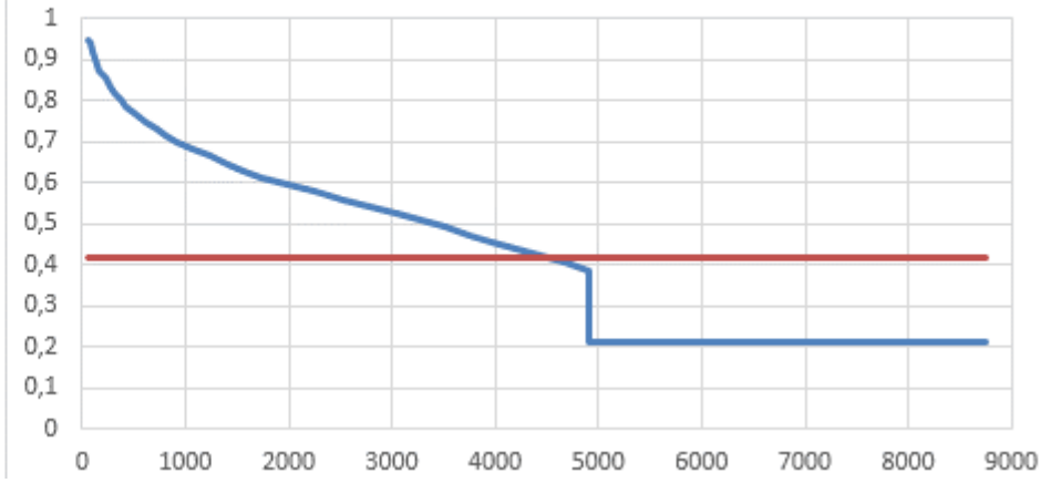
Рисунок 2.5 - График Россандера с. Покровское ДОХБ
