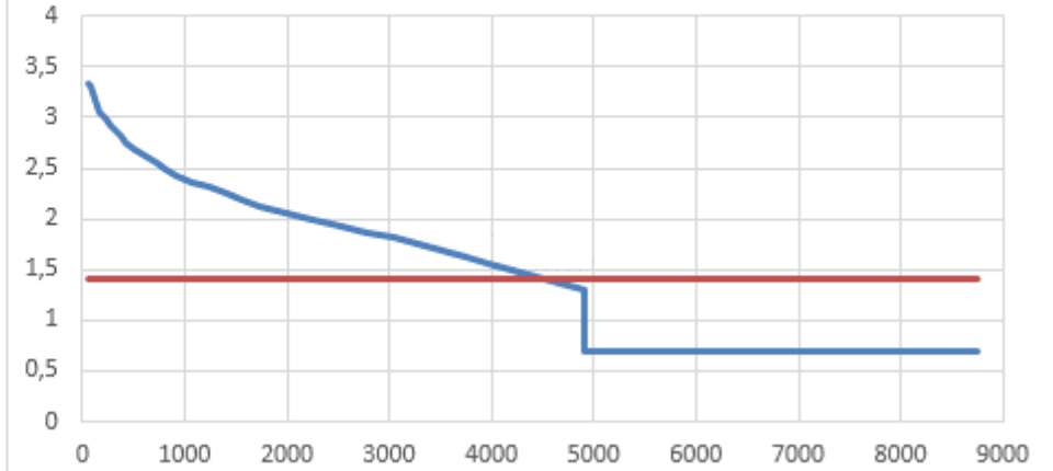
Рисунок 2.4 - График Россандера котельной д. Нововолково
