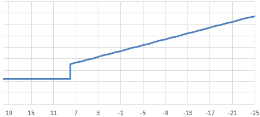
Рисунок 2.6 - График Россандера котельной с. Покровское ЖКХ
