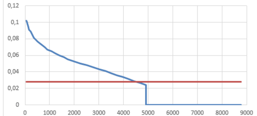
Рисунок 2.9 - График Россандера котельной д. Городище
