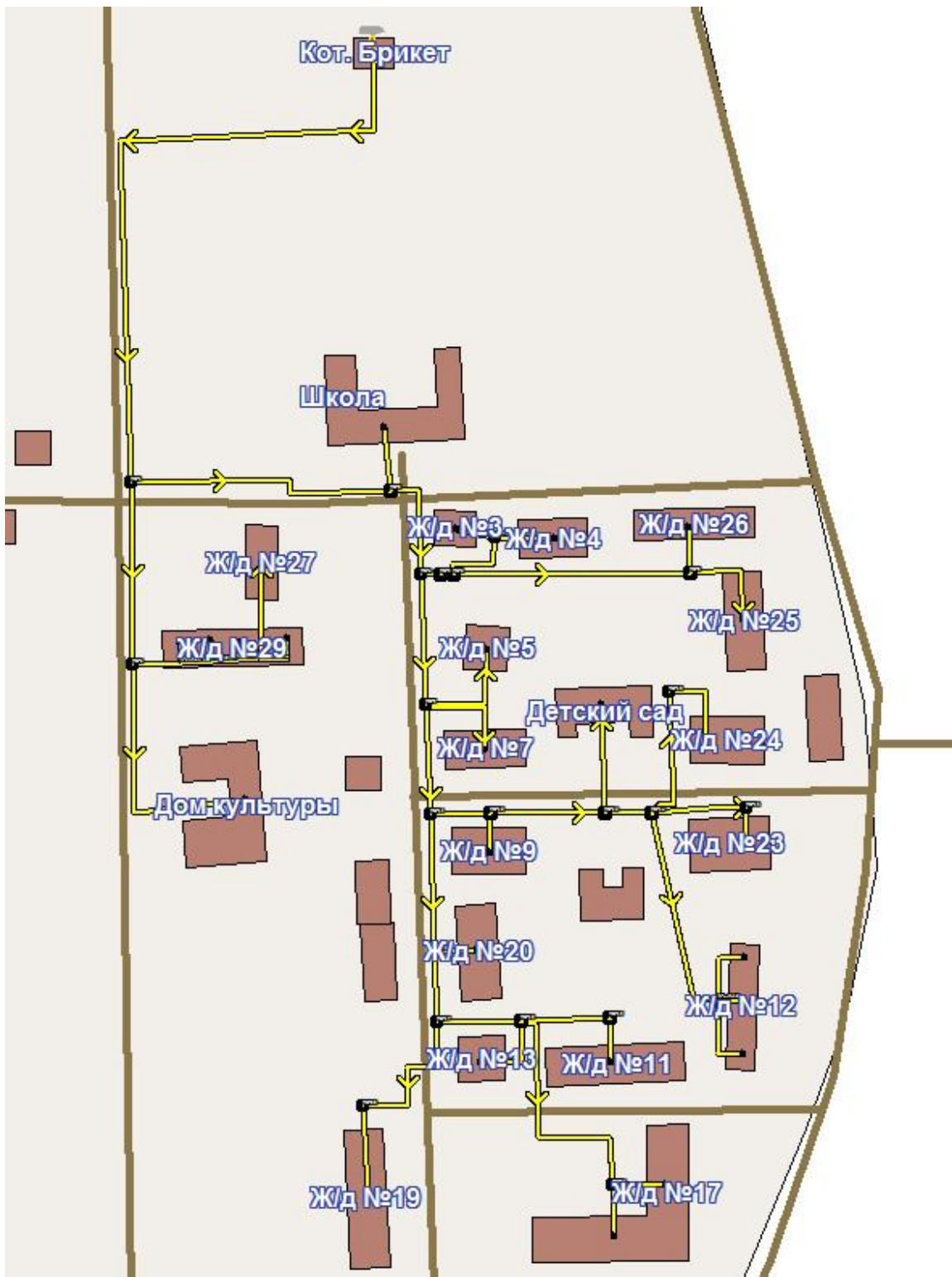
Рисунок 3.8 - Схема тепловой сети котельной п. Брикет
