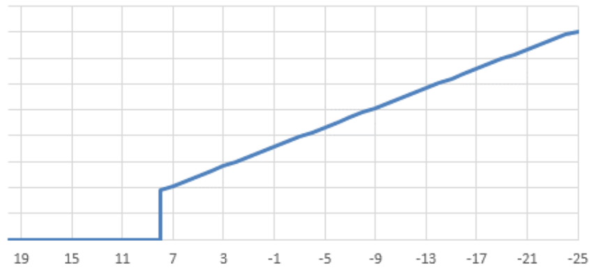
Рисунок 2.7 - График Россандера котельной д. Ивойлово
