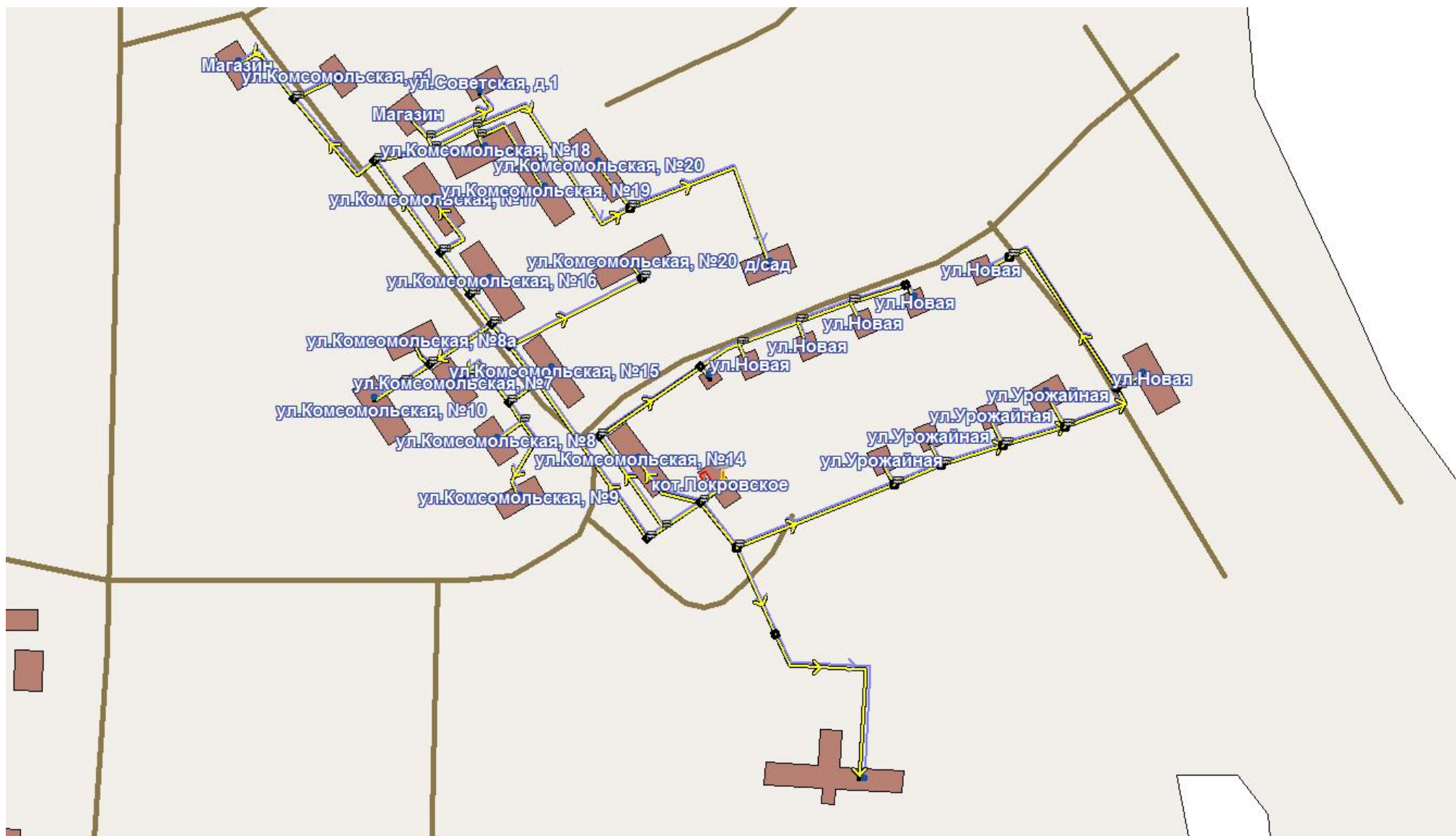
Рисунок 3.3 - Схема тепловой сети котельной с. Покровское, ЖКХ
