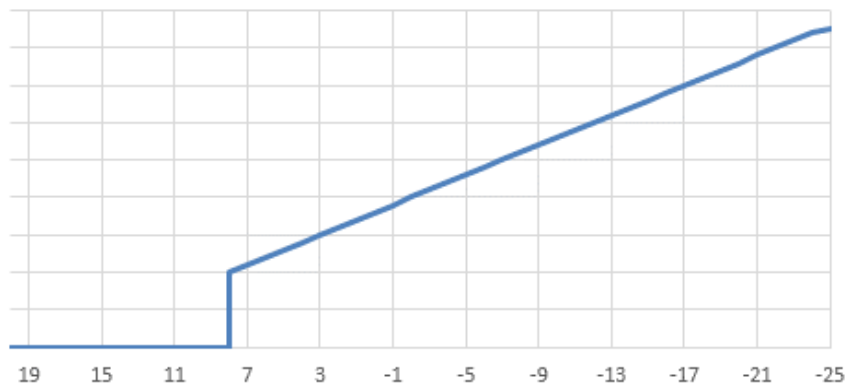
Рисунок 2.11 - График Россандера котельной п. Брикет
