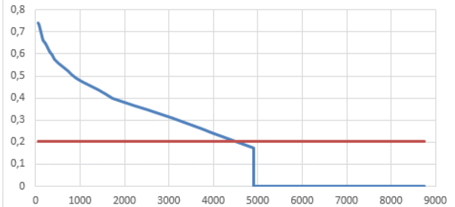
Рисунок 2.8 - График Россандера котельной в/ч «Ольховка»
