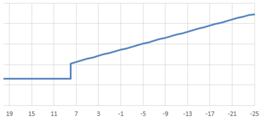
Рисунок 2.10 - График Россандера котельной с. Никольское
