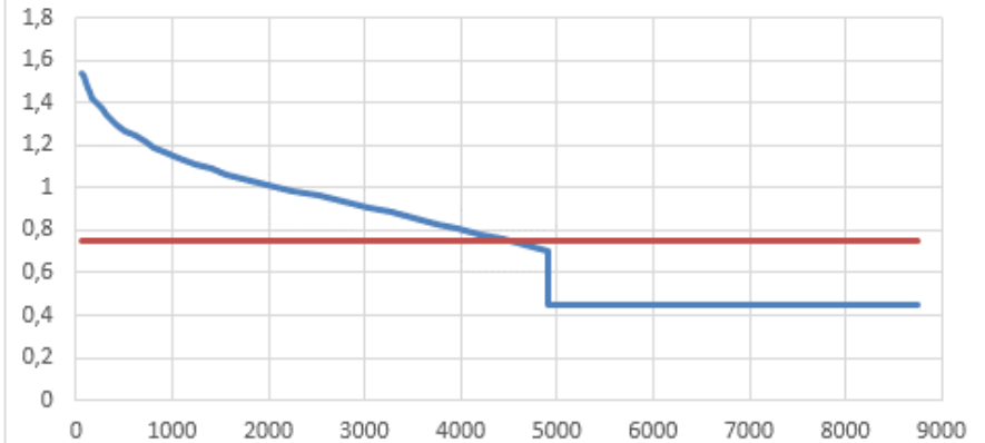
Рисунок 2.6 - График Россандера котельной с. Покровское ЖКХ
