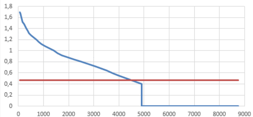
Рисунок 2.11 - График Россандера котельной п. Брикет
