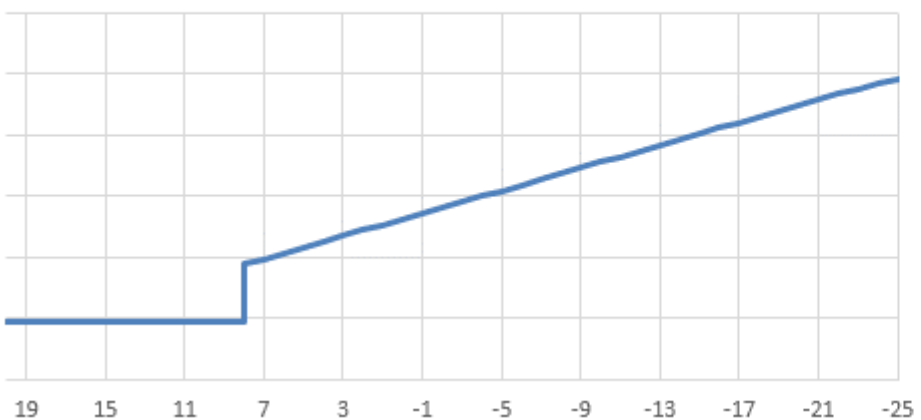
Рисунок 2.5 - График Россандера котельной д. Воробьево
