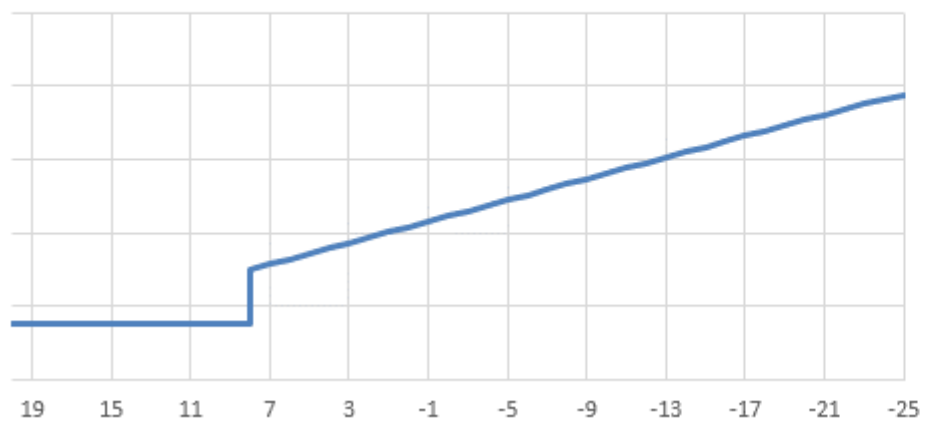
Рисунок 2.12 - График Россандера котельной д. Сытьково
