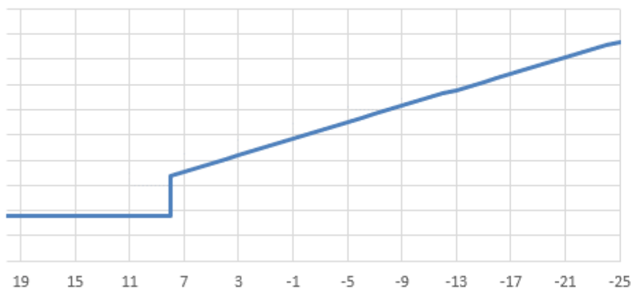
Рисунок 2.4 - График Россандера котельной д. Нестерово
