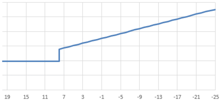
Рисунок 2.8 - График Россандера котельной п. Новотеряево
