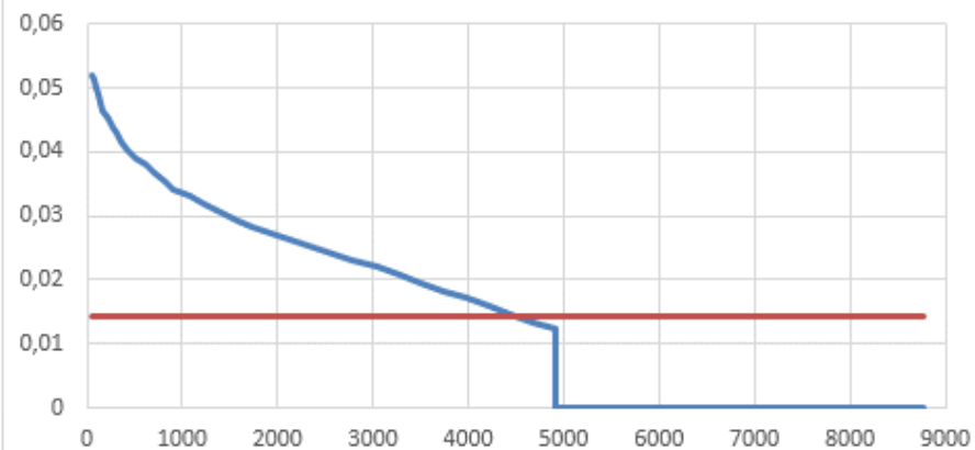
Рисунок 2.10 - График Россандера котельной д. Ватулино
