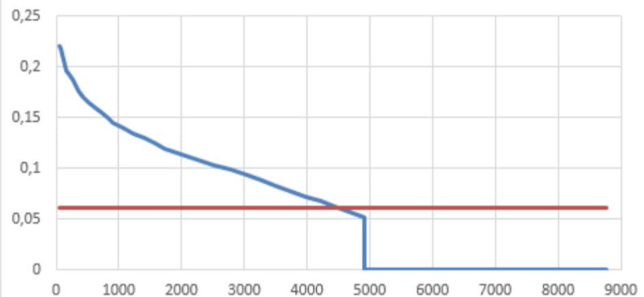
Рисунок 2.9 - График Россандера котельной д. Костино
