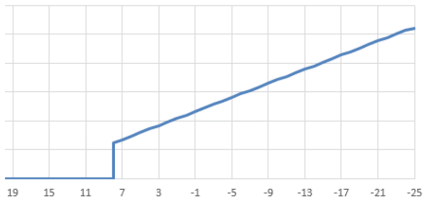
Рисунок 2.10 - График Россандера котельной д. Ватулино
