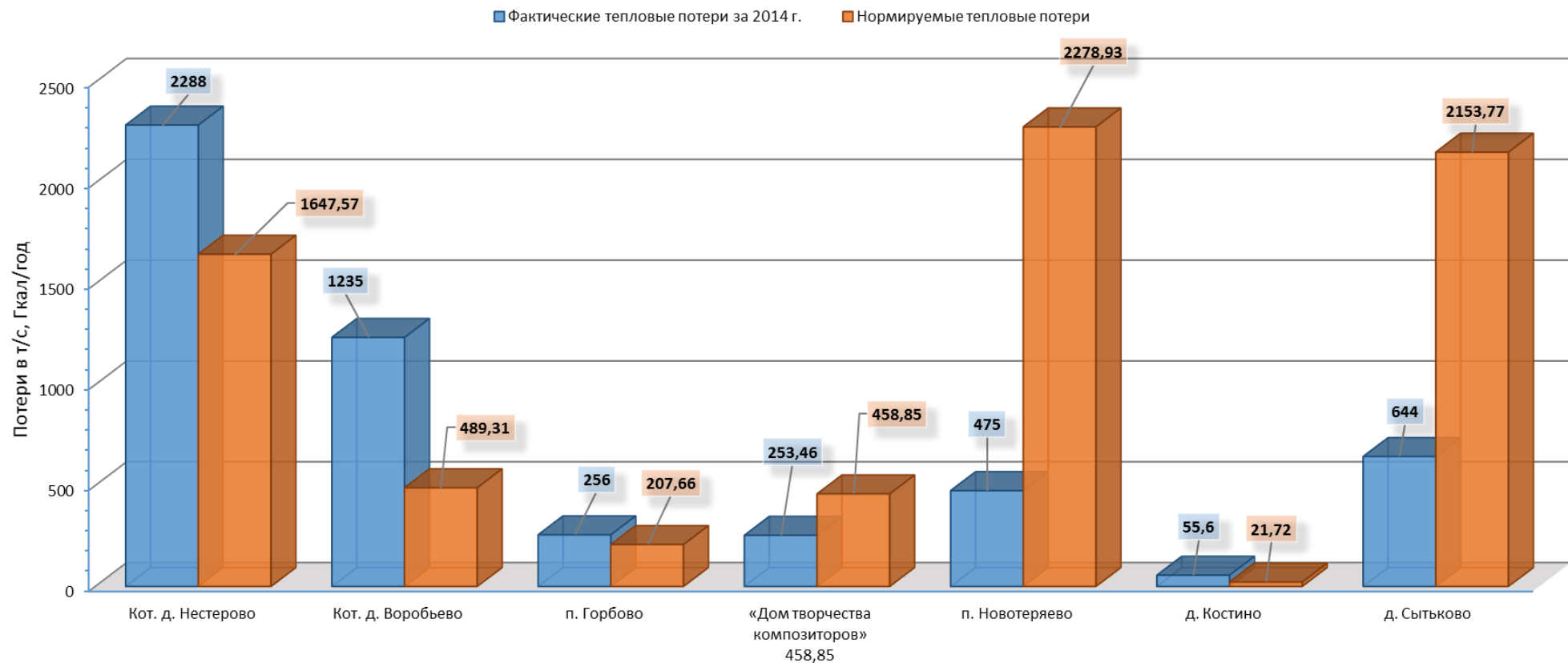
Рисунок 3.9 - Потери в тепловых сетях котельных сельского поселения Староружское
