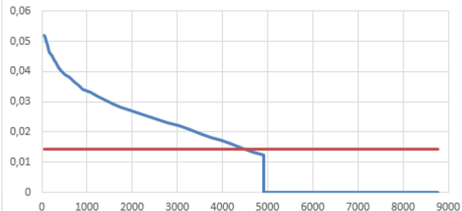
Рисунок 2.11 - График Россандера котельной д. Комлево
