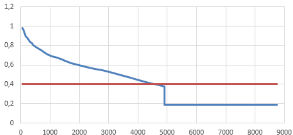
Рисунок 2.5 - График Россандера котельной д. Воробьево
