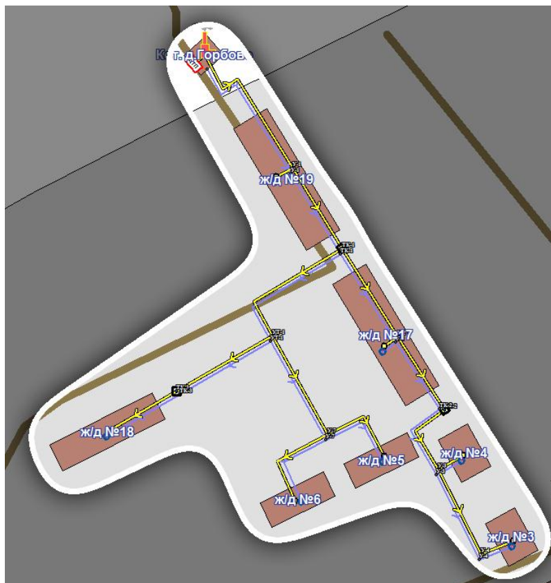
Рисунок 4.3 - Зона действия системы теплоснабжения котельной п. Горбово сельского поселения Старорусское
