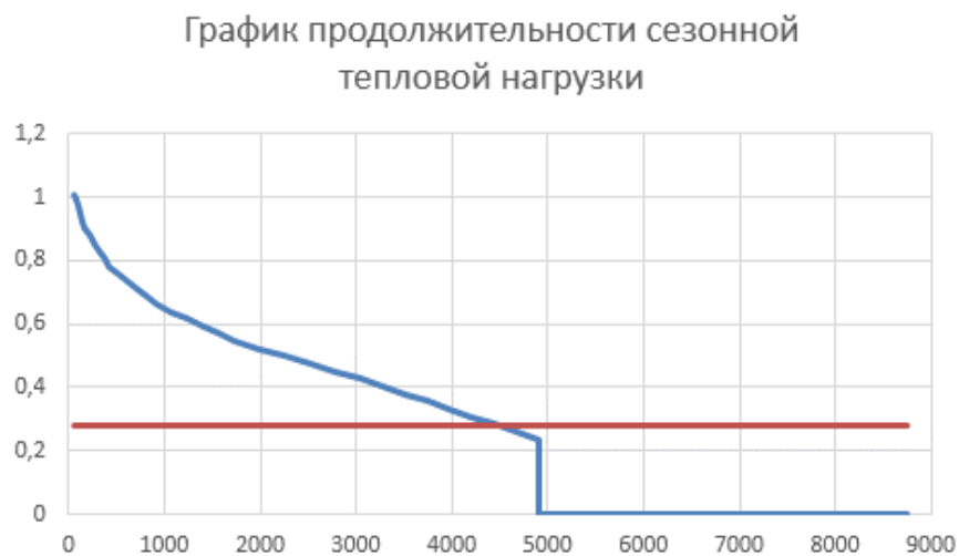
Рисунок 2.7 - График Россандера котельной «Дом творчества композиторов»
