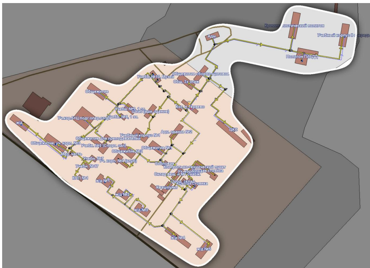
Рисунок 4.5 - Зона действия системы теплоснабжения котельной п. Новотеряево сельского поселения Старорузское
