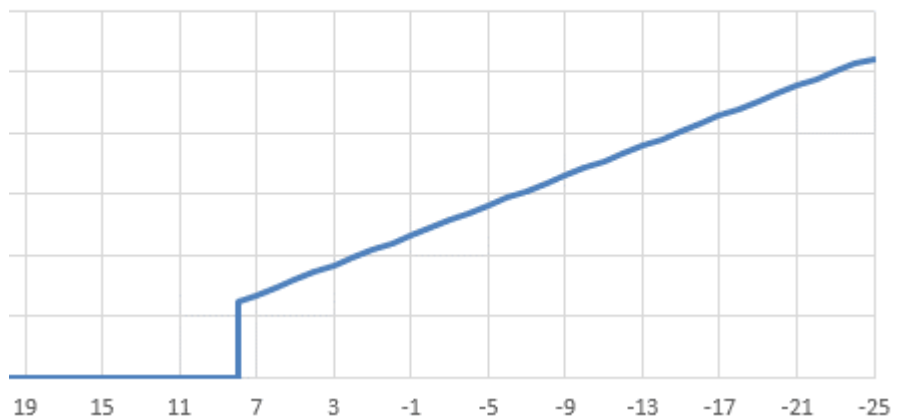
Рисунок 2.11 - График Россандера котельной д. Комлево
