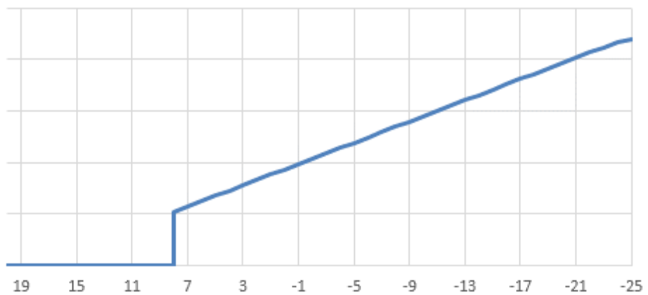
Рисунок 2.9 - График Россандера котельной д. Костино
