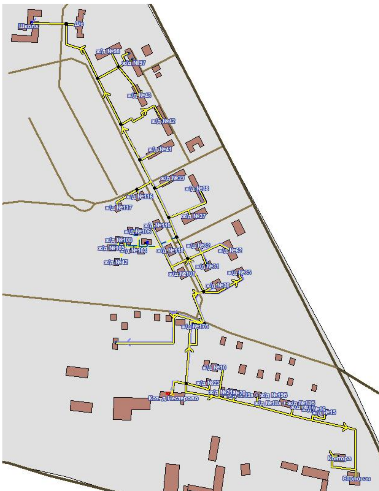
Рисунок 3.1 - Схема тепловой сети котельной д. Нестерово
