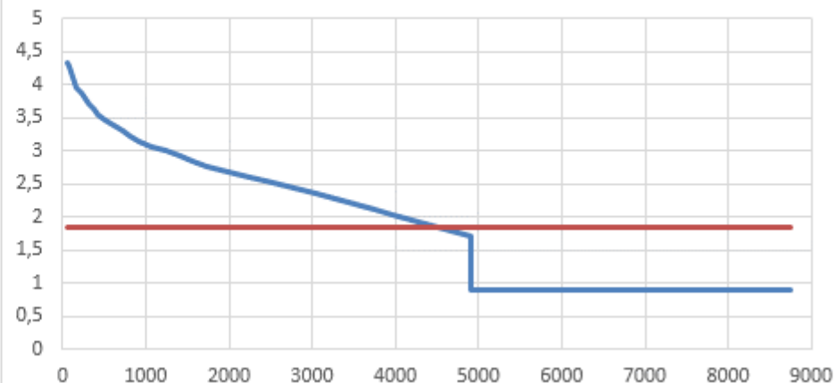
Рисунок 2.4 - График Россандера котельной д. Нестерово
