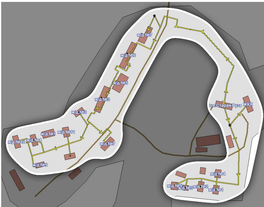
Рисунок 4.4 - Зона действия системы теплоснабжения котельной «Дом творчества композиторов» сельского поселения Старорузское
