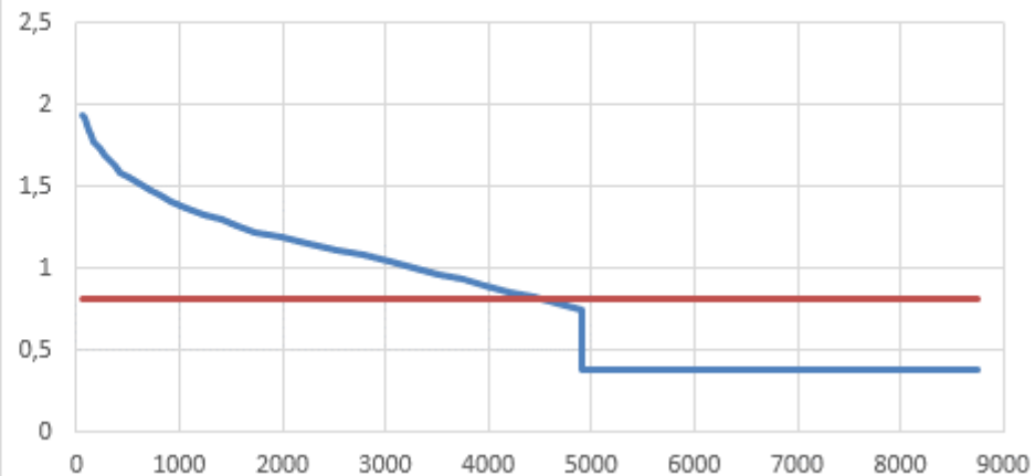
Рисунок 2.12 - График Россандера котельной д. Сытьково
