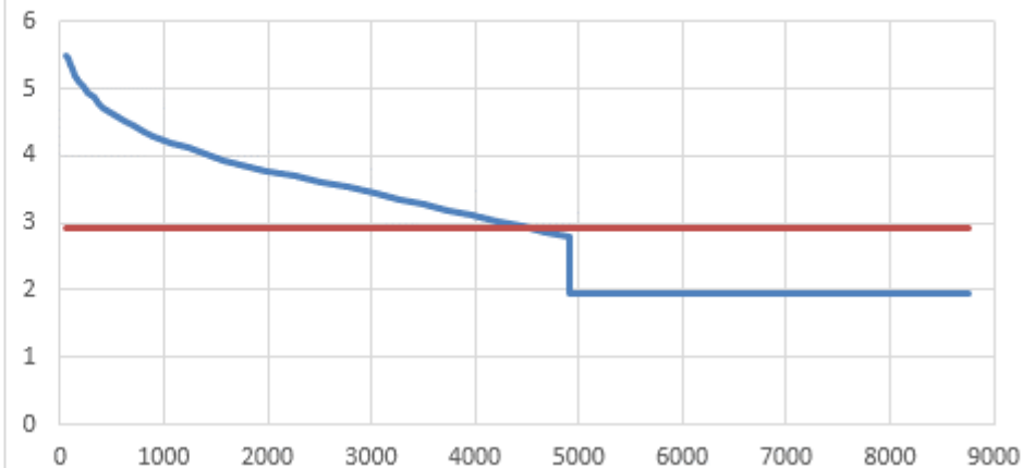
Рисунок 2.8 - График Россандера котельной п. Новотеряево
