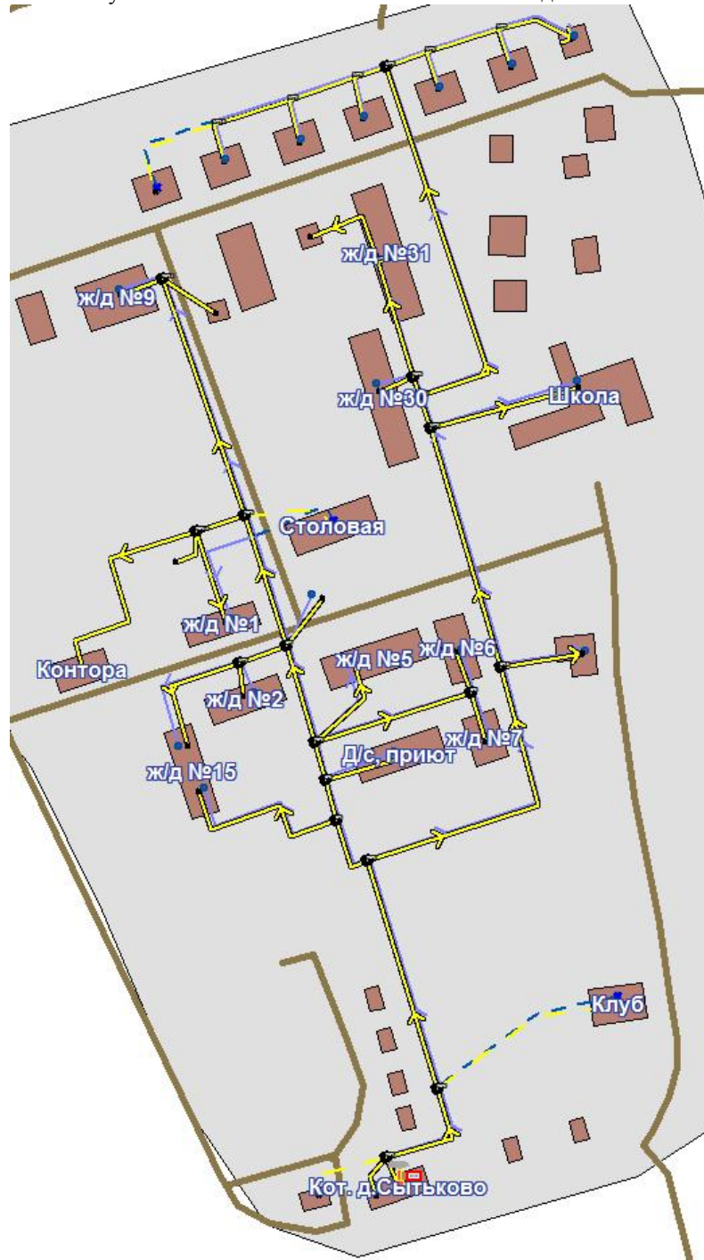
Рисунок 3.7 - Схема тепловой сети котельной д. Сытьково
