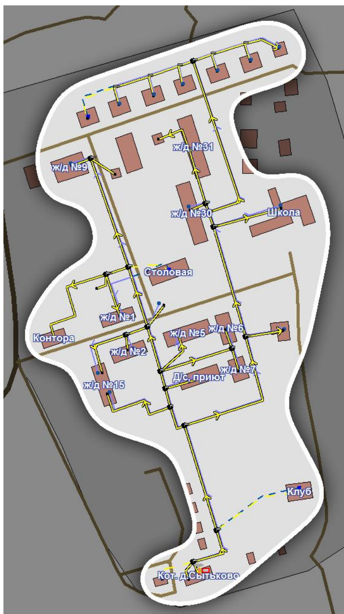
Рисунок 4.7 - Зона действия системы теплоснабжения котельной д. Сытьково сельского поселения Старорусское
